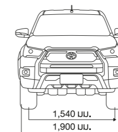
ไฮลักซ์ รีโว่ ร็อคโค รุ่นสมาร์ท แค็บ พรินเนออร์ ขับเคลื่อน 2 ล้อ ยกสูง 2.4 AT สี PLATINUM WHITE PEARL
