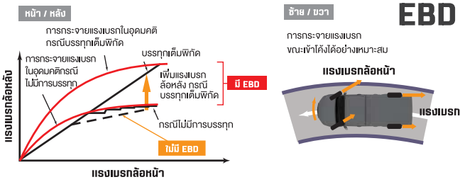
ระบบกระจายแรงเบรก EBD (Electronic Brake-force Distribution)
