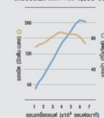
เครื่องยนต์ 2ZR-FBE 1,800 ซีซี
