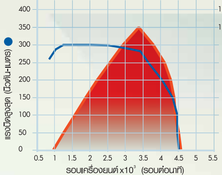
เครื่องยนต์ 1KD-FTV
