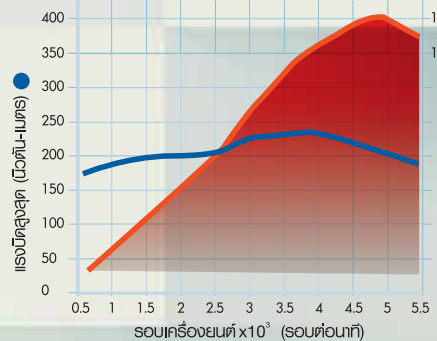
เครื่องยนต์ 2TR-FE
